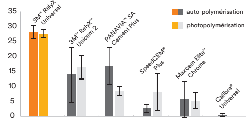
Résistance du collage au cisaillement (MPa) sur dentine après un vieillissement artificiel
